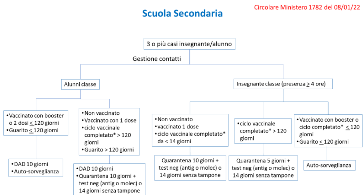
Figura 3. Scuola secondaria con 3 o più casi
